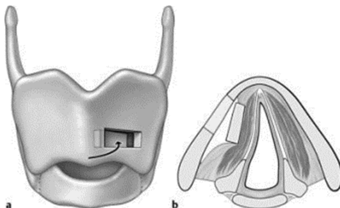
Figuur 1: Schematische tekening van het schildkraakbeen (de adamsappel).
