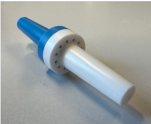
Afbeelding: Ontluchttingsdopje- de blauwe kant sluit u aan op de maaghevel.
